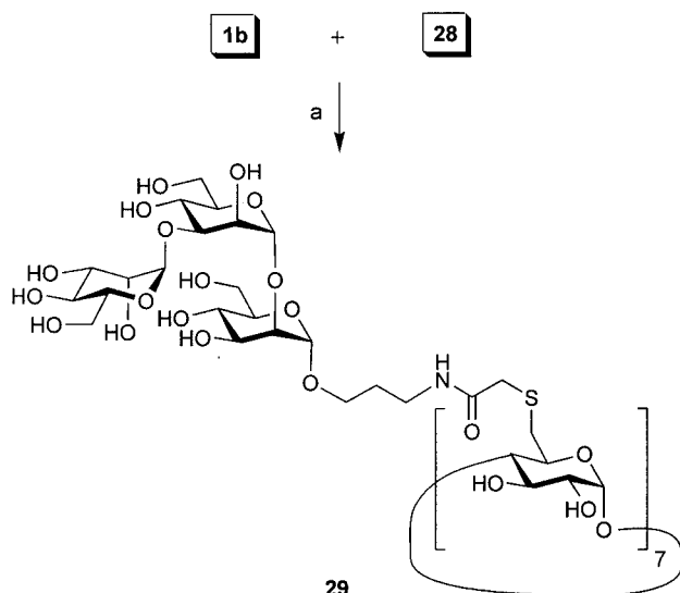
Scheme 4. a) \text{K}_2\text{CO}_3 , DMF/ \text{H}_2\text{O} , 9:1, 54%.
